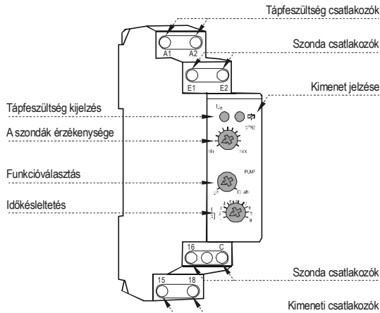
NIVOCONT KRK-512-5 előlapja a kezelőszervekkel
