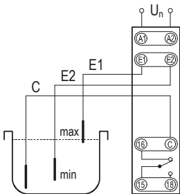
NIVOCONT KRK-512-5 bekötése
